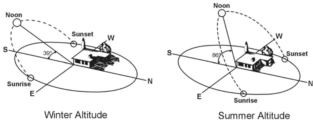
Figure 5. Sun Path Diagrams for 28° N. Latitude
